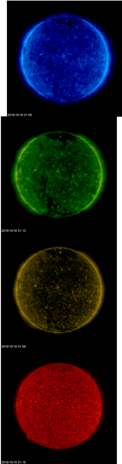
EIT 171
